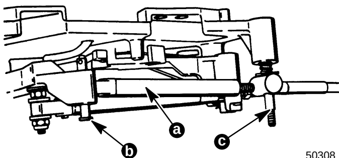
a - Remote Control Shift Cable b - Clevis Pin c - Stud
